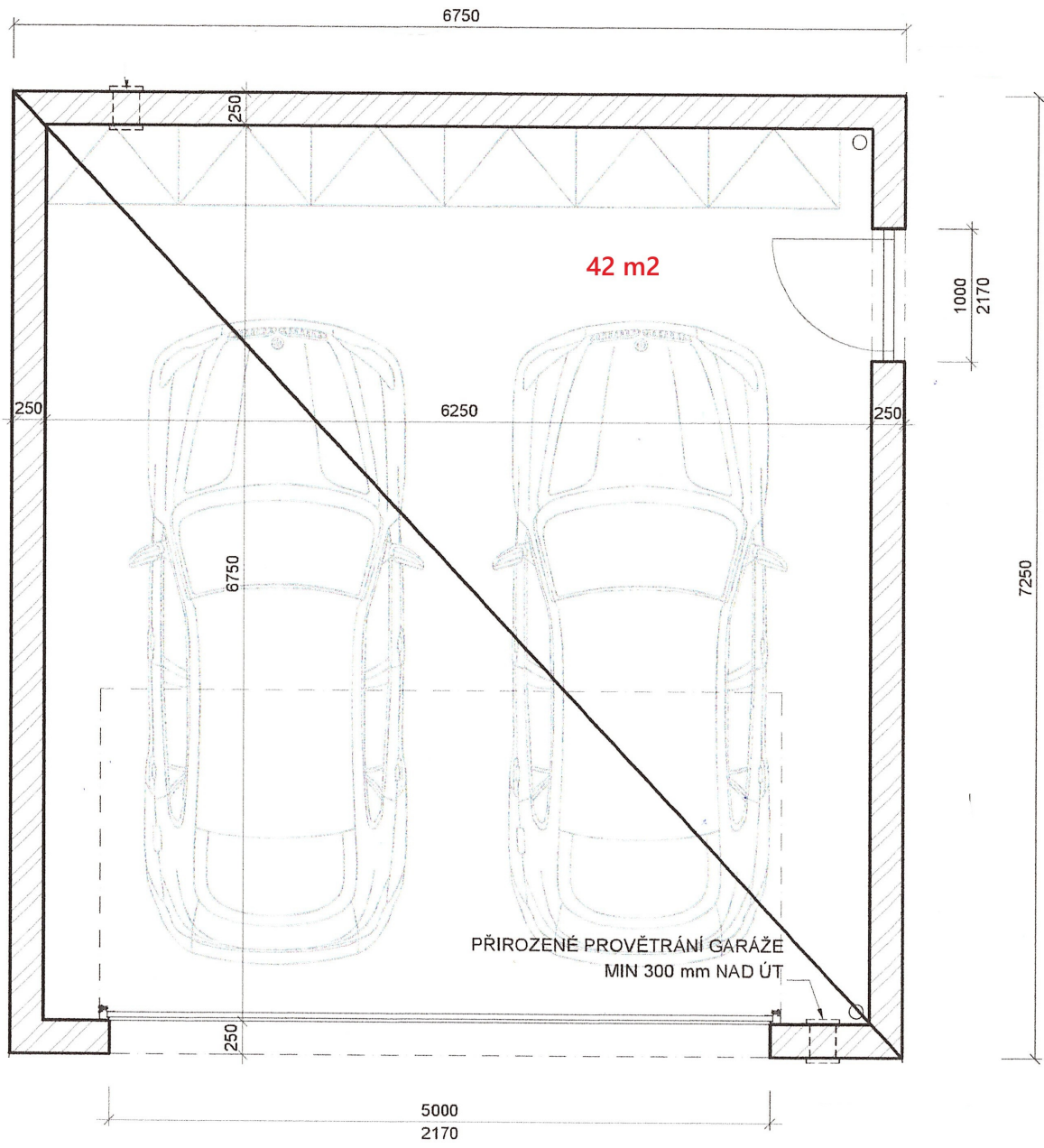
Půdorys - garáž
